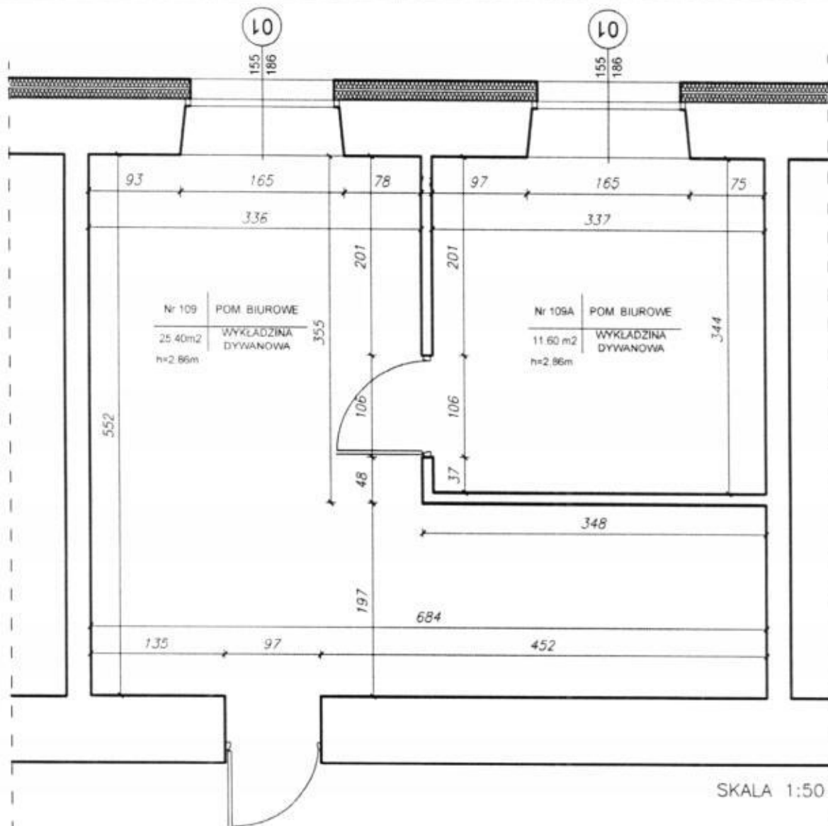
RZUT PIĘTRA POMIESZCZENIE NR 109
