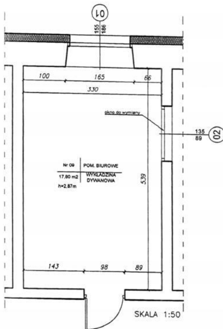
RZUT PARTERU POMIESZCZENIE NR 9
