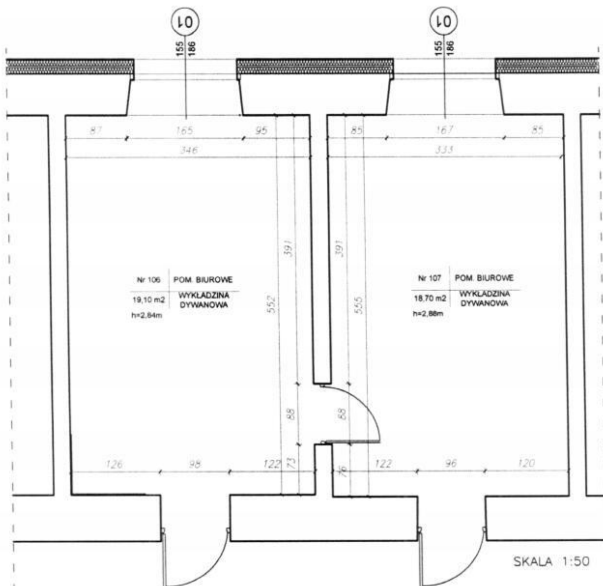
RZUT PIĘTRA POMIESZCZENIE NR 106
