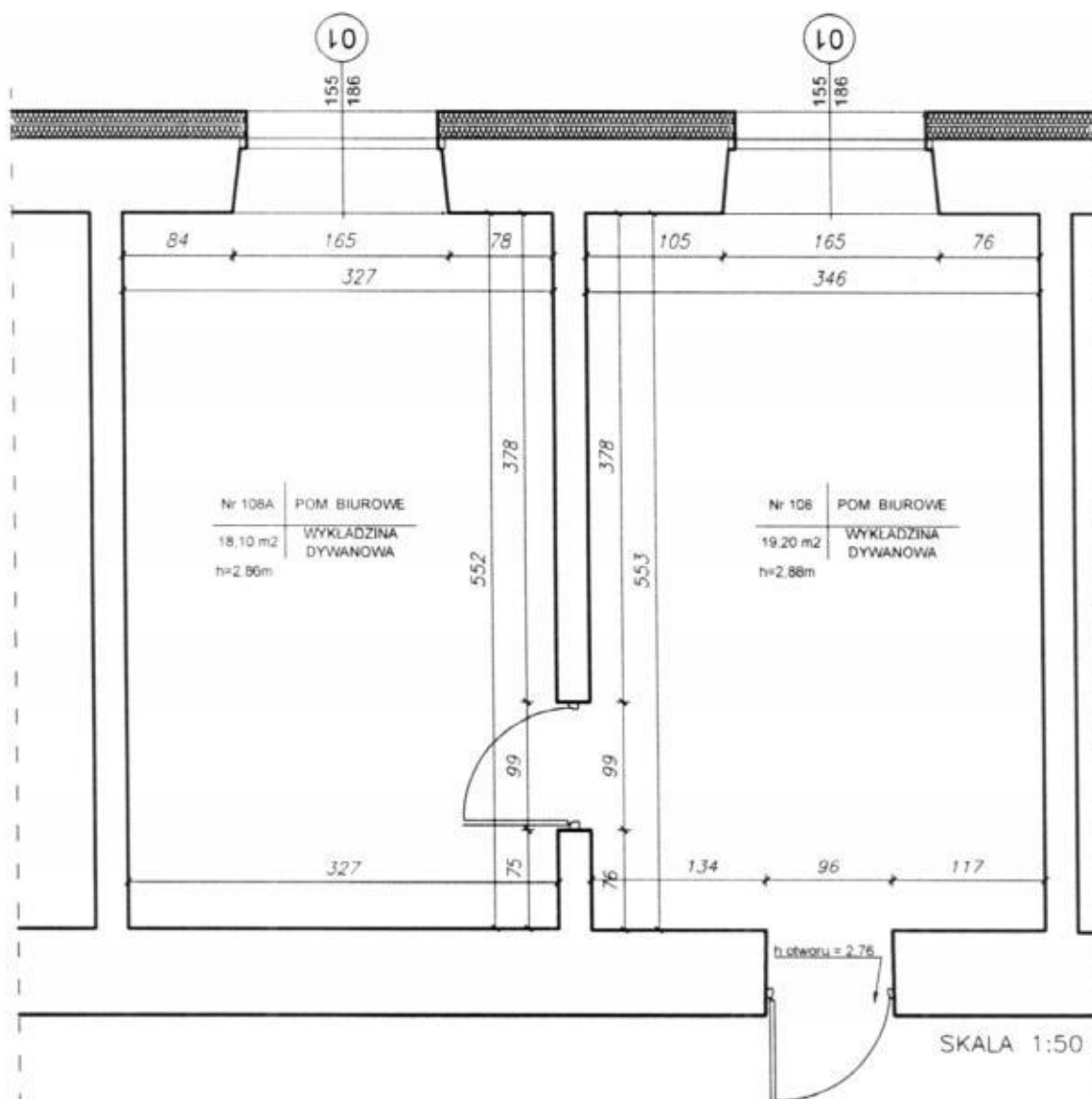
RZUT PIĘTRA POMIESZCZENIE NR 108A
